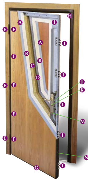
Voorbeeld van een deurblok met een a2p BP 3-certificaat
